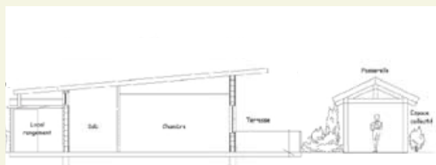
Coupe sur maison du résident(plan non contractuel)
